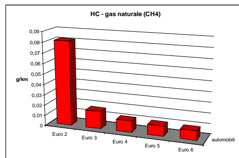
Fattori di emissione per veicoli bifuel a metano – Idrocarburi totali (HC) a 50 Km/h a 90 Km/h
