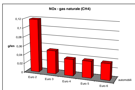
Fattori di emissione per veicoli bifuel a metano – Ossidi di azoto (NO x ) a 50 Km/h a 90 Km/h
