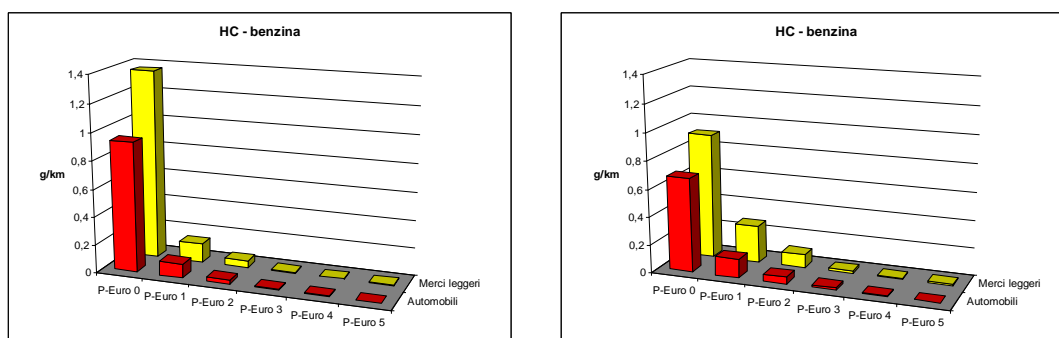
a 50 Km/h a 90 Km/h Fattori di emissione per veicoli a benzina - Idrocarburi totali (HC)
