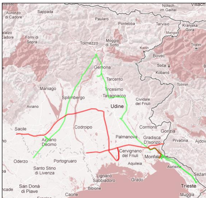
Rappresentazione della rete di trasmissione dell'energia elettrica a 220 kV (verde) e 380 kV (rosso).
