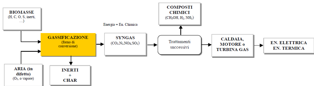
Schematizzazione del processo di gassificazione (fonte: Whiting, 1998)
