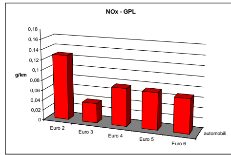
Fattori di emissione per veicoli bifuel a GPL – Ossidi di azoto (NOx) a 50 Km/h a 90 Km/h
