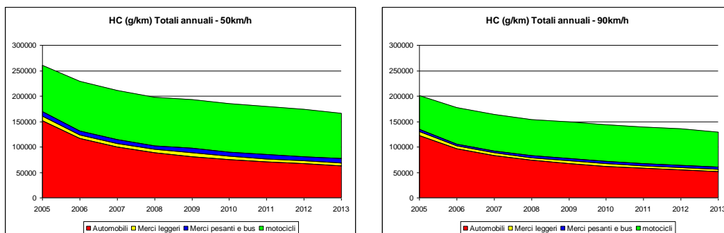
Idrocarburi totali (HC):emissioni complessive del parco veicolare per km a 50 Km/h a 90 Km/h
