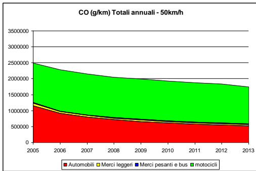
Ossido di Carbonio (CO): emissioni complessive del parco veicolare per km a 50 Km/h a 90 Km/h
