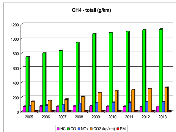
Emissione annuale per chilometro per l'intero parco circolante bifuel a Metano a 50 Km/h
