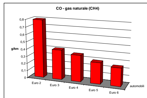
Fattori di emissione per veicoli bifuel a metano – Monossido di carbonio (CO) a 50 Km/h a 90 Km/h
