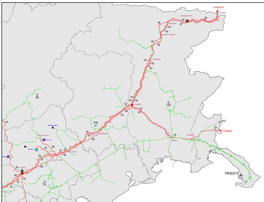
Rete Snam nel Nord-Est Italia - Fonte: Snam Rete Gas.
