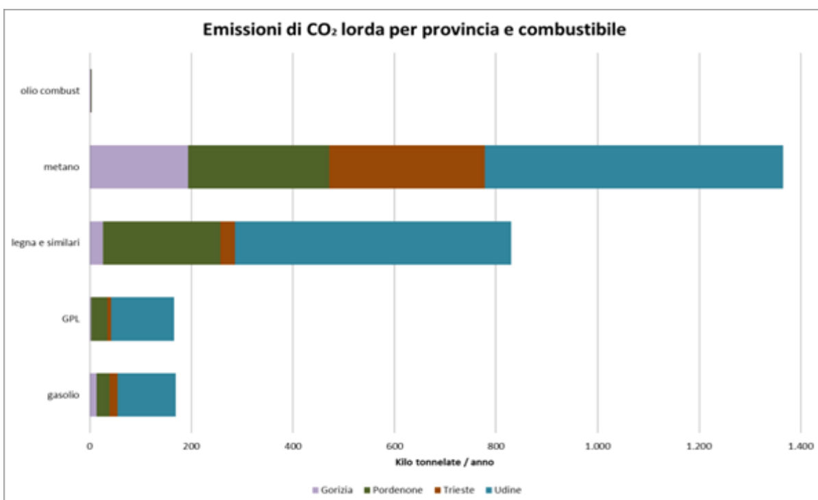
Emissioni dei principali inquinanti (inclusa il CO 2 lordo) associate ai diversi vettori energetici usati in ambito domestico e commerciale
