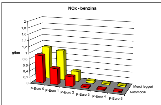
a 50 Km/h a 90 Km/h Fattori di emissione per veicoli a benzina – Ossidi di azoto (NO x )
