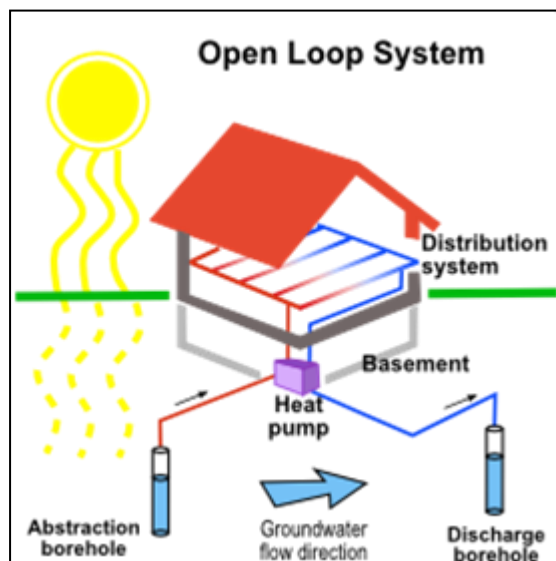
Impianto geotermico a bassa entalpia a ciclo aperto, detto anche: impianto "idrotermico"
