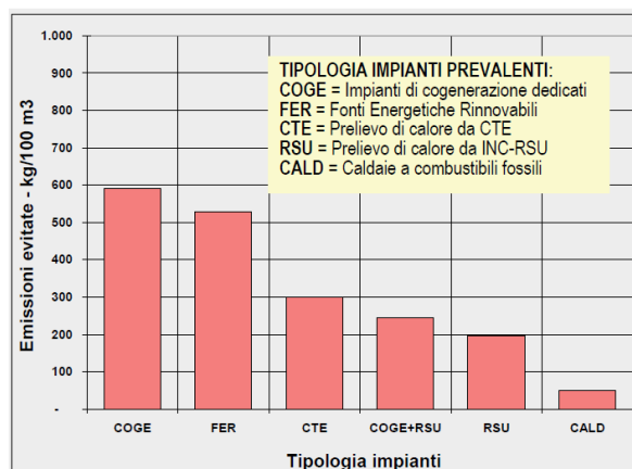
Emissioni evitate di CO 2 dai sistemi di teleriscaldamento in funzione della tecnologia prevalente del sistema di produzione dell'energia - Fonte: ENEA 2008 -
