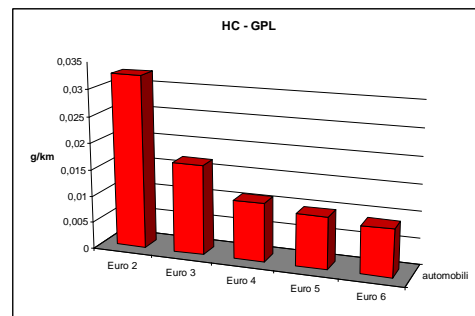
Fattori di emissione per veicoli bifuel a GPL – Idrocarburi totali (HC) a 50 Km/h a 90 Km/h
