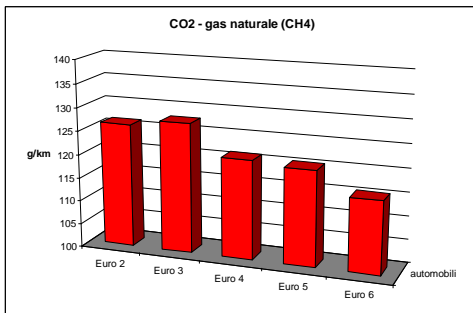
Fattori di emissione per veicoli bifuel a metano – Biossido di carbonio (CO 2 ) a 50 Km/h a 90 Km/h
