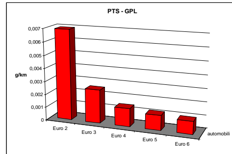
Fattori di emissione per veicoli bifuel a GPL – Particolato totale (PTS) a 50 Km/h a 90 Km/h
