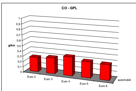
Fattori di emissione per veicoli bifuel a GPL – Monossido di carbonio (CO) a 50 Km/h a 90 Km/h
