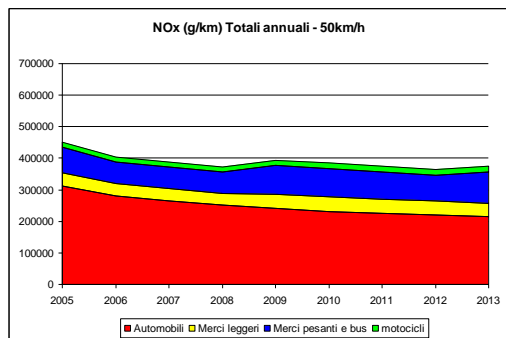
Ossidi di Azoto (NO x ): emissioni complessive del parco veicolare per km a 50 Km/h a 90 Km/h
