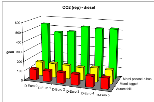
a 50 Km/h a 90 Km/h Fattori di emissione per veicoli Diesel – Biossido di carbonio (CO 2 )
