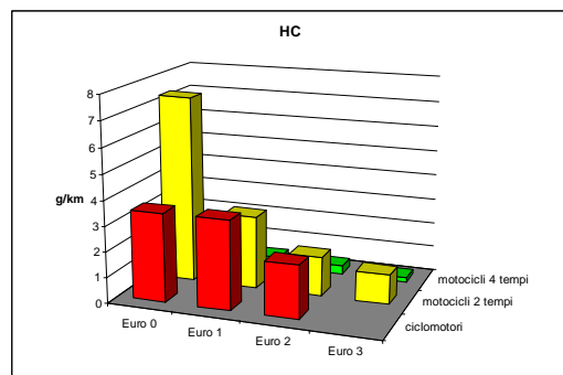
a 50 Km/h a 90 Km/h Fattori di emissione per soli motocicli - Idrocarburi totali (HC)
