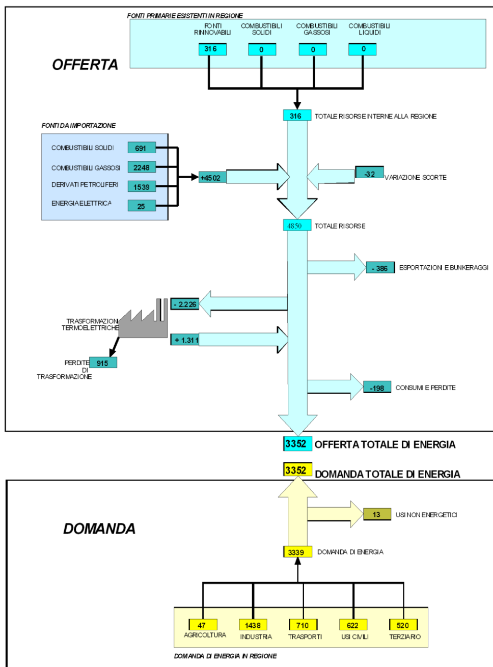
Schema semplificato del sistema energetico regionale al 2008
