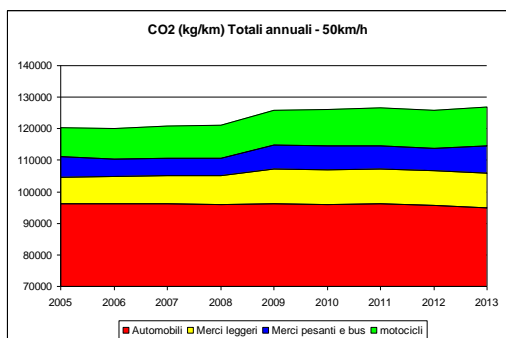
Biossido di Carbonio (CO 2 ): emissioni complessive del parco veicolare per km
