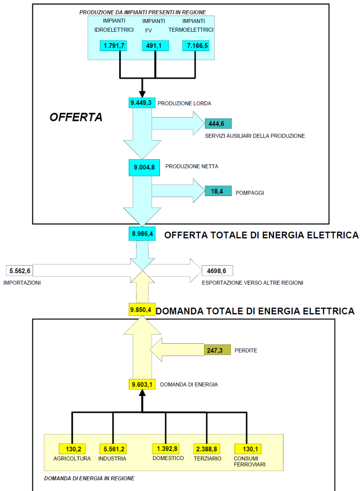
Bilancio elettrico regionale per l'anno 2013 (valori in GWh) Fonte: Rielaborazione dati TERNA, Dati statistici Bilanci elettrici regionali 2013
