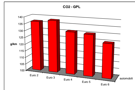
Fattori di emissione per veicoli bifuel a GPL – Biossido di carbonio (CO 2 ) a 50 Km/h a 90 Km/h
