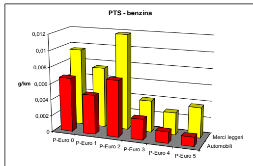
a 50 Km/h a 90 Km/h Fattori di emissione per veicoli a benzina – Particolato totale (PTS)
