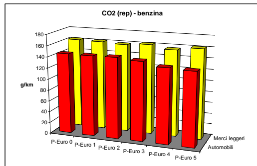
a 50 Km/h a 90 Km/h Fattori di emissione per veicoli a benzina – Biossido di carbonio (CO 2 )
