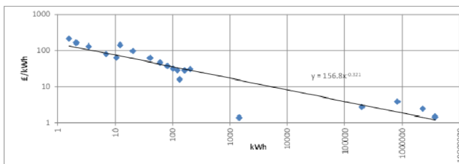
Andamento del costo dello stoccaggio dell'acqua calda (£/KWh) - Fonte: Mark Barrett 2012. UCL Energy Institute, London
