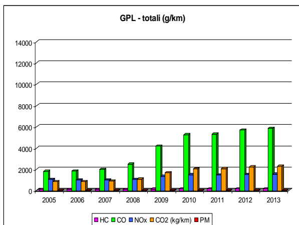
Emissione annuale per chilometro - per l'intero parco circolante bifuel a GPL
