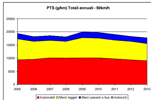
Materiale Particolato totale (PTS): emissioni complessive del parco veicolare per km a 50 Km/h a 90 Km/h
