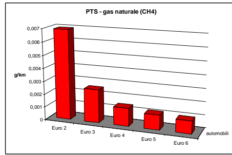
Fattori di emissione per veicoli bifuel a metano – Particolato totale (PTS) a 50 Km/h a 90 Km/h
