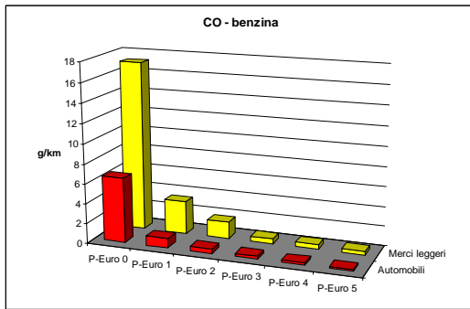
a 50 Km/h a 90 Km/h Fattori di emissione per veicoli a benzina – Monossido di carbonio (CO)
